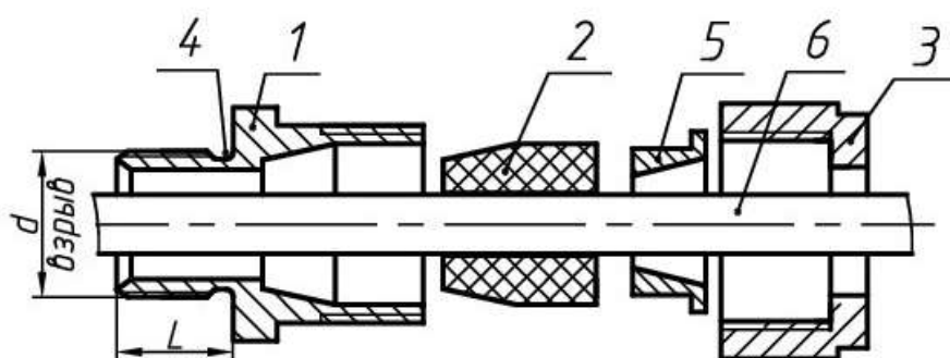
Рис. В.3.б – Порядок сборки кабельного ввода К для открытой прокладки небронированного кабеля:
