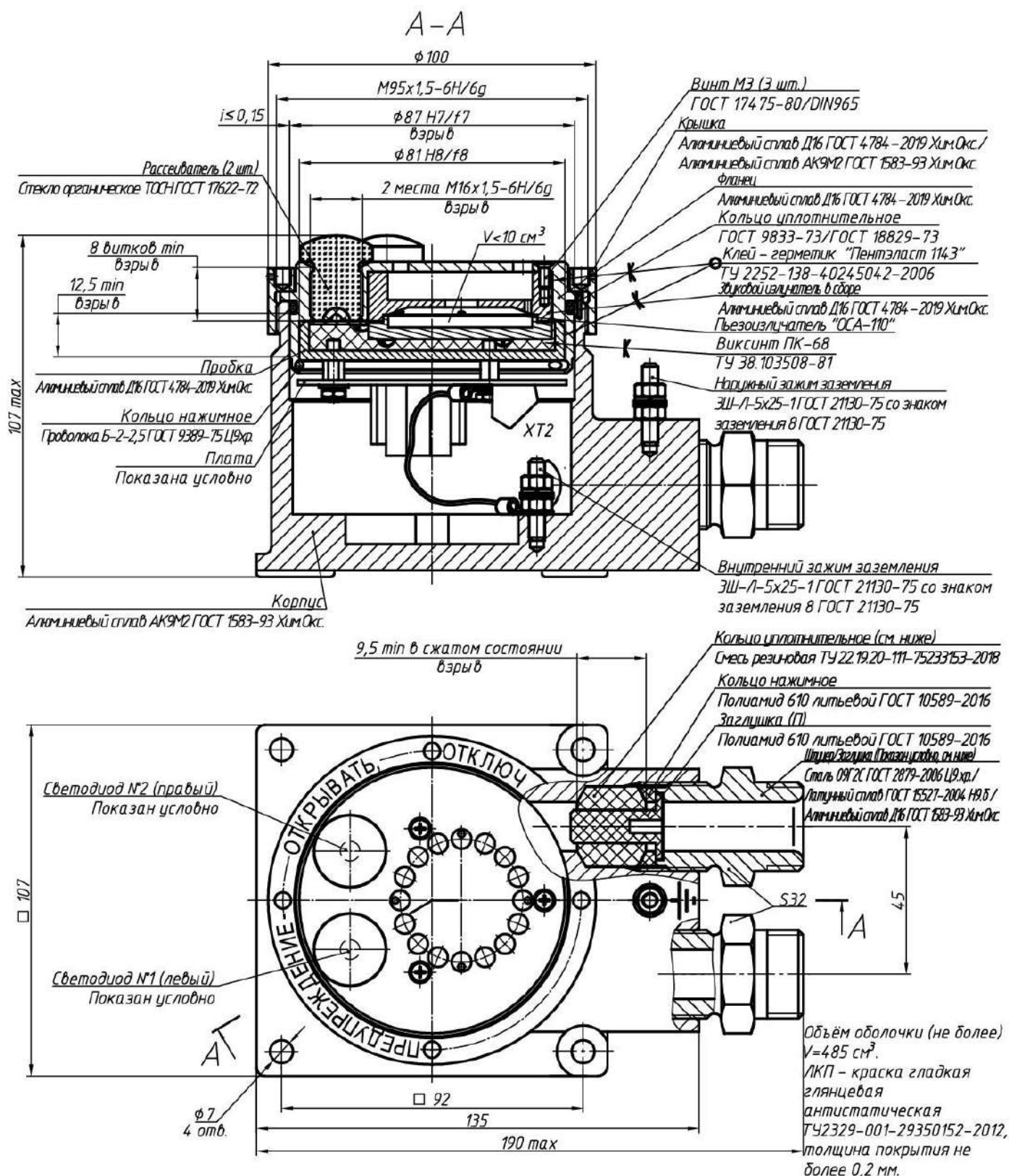
Рис. А.2.б - Габаритный чертёж оповещателей моделей ЕхОПЗС-А в корпусе из алюминиевого сплава, совмещённый с чертежом взрывозащиты. Монтаж кабеля диаметром от 8 до 18 мм. Кабельные входы ЗАО НПК ЭТАЛОН см на рис. А.3 – А.15 приложения А. Маркировка показана в п. 1.6.
