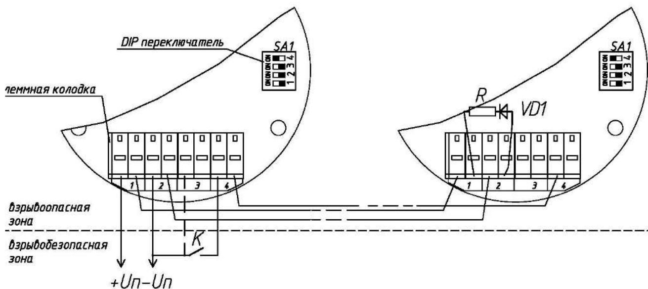
Рис.Б.4.а Схема подключения нескольких светозвуковых оповещателей ЕхОПЗС с индексом 220 для работы в режимах 1 (контакт К разомкнут) и 2 (контакт К замкнут). Звуковой сигнал оповещателей выбирается переключателями SA1.1, SA1.2 (см. таблицу Б.1 выше), световой сигнал светодиодов 1 и 2 оповещателей выбирается переключателями SA1.3, SA1.4 (см. таблицу Б.2 выше). При наличии переключателя SA1.5 см также таблицу Б.3
