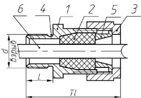
Рис. В.3.а - Кабельные вводы ВВКм (условное обозначение К ) для открытой прокладки кабеля, размеры см. в таблице В.3
