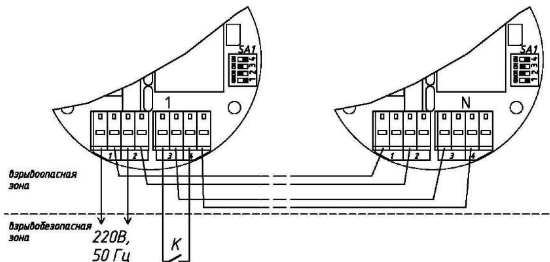
Рис.Б.4.а Схема подключения нескольких светозвуковых оповещателей ЕхОПЗС с индексом 220 для работы в режимах 1 (контакт К разомкнут) и 2 (контакт К замкнут). Звуковой сигнал оповещателей выбирается переключателями SA1.1, SA1.2 (см. таблицу Б.1 выше), световой сигнал светодиодов 1 и 2 оповещателей выбирается переключателями SA1.3, SA1.4 (см. таблицу Б.2 выше). При наличии переключателя SA1.5 см также таблицу Б.3
