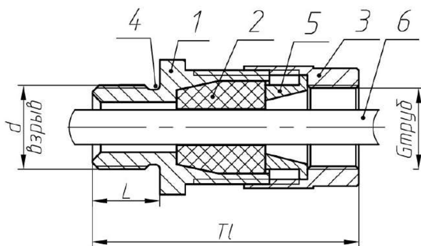
Рис. В.4.а - Кабельные вводы ТВВКм (условное обозначение Т ) для прокладки кабеля в трубе с наружной резьбой. Размеры см. в таблице В.4.
