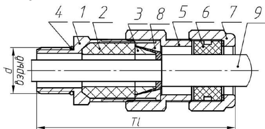
Рис. В.2.а – Кабельный ввод АВВКм (условное обозначение БСЗ ) для монтажа бронированного кабеля с заземлением брони, размеры см. в таблице В.2
