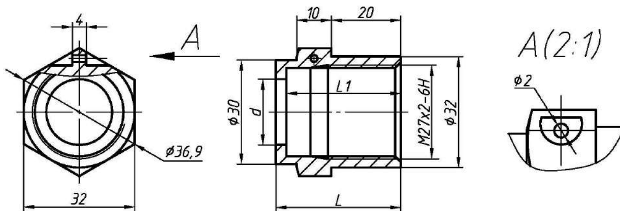
Рис. А. 12 – Кожух БСЗ. Размеры см в таблице А.6
