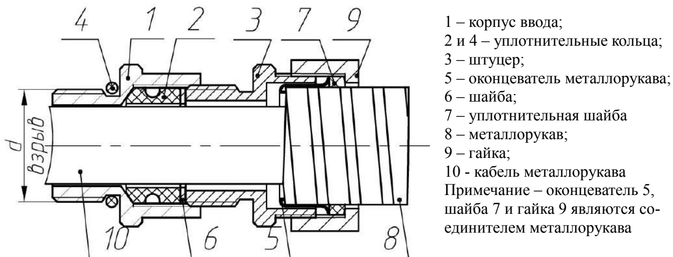
Рис. В.1.а – Кабельный ввод СВВКм (условное обозначение М ) для прокладки кабеля в металлорукаве, размеры см. в таблице В.1
