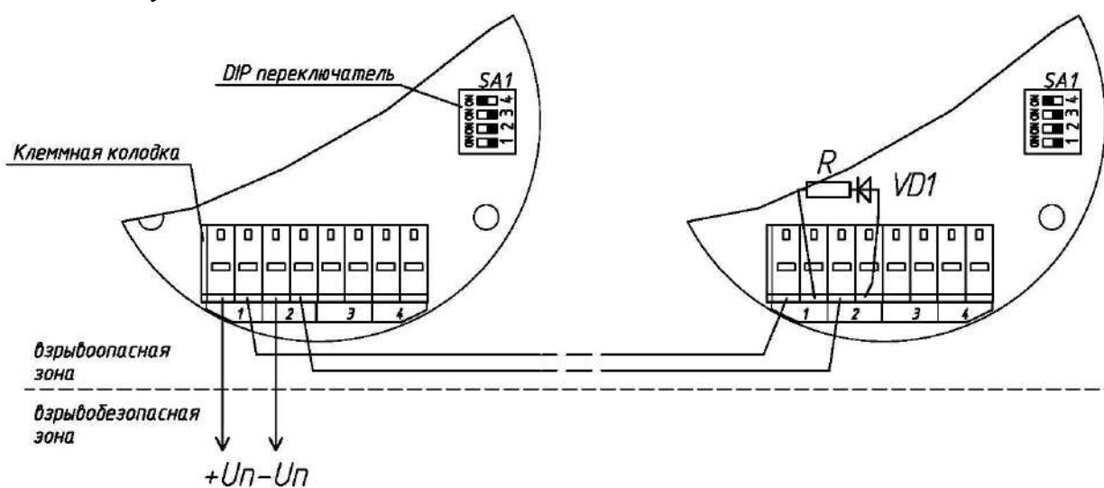
Рис. Б.3.а Схема подключения нескольких светозвуковых оповещателей ЕхОПЗС с индексом 220 для работы в режиме 1. Звуковой сигнал оповещателей выбирается переключателями SA1.1, SA1.2 (см. таблицу Б.1 выше), световой сигнал светодиода 1 оповещателей выбирается переключателями SA1.3, SA1.4 (см. таблицу Б.2 выше). При наличии переключателя SA1.5 см также таблицу Б.3
